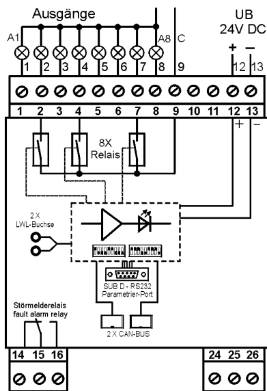
Grundmodul mit LWL-Modem und 8 Ausgangsrelais
