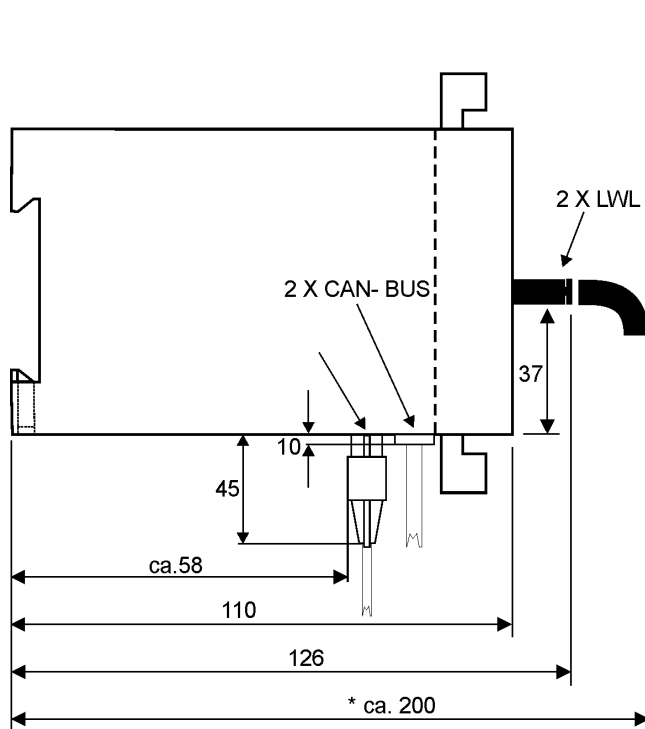
Grundmodul mit LWL-Modem und 8 Ausgangsrelais
