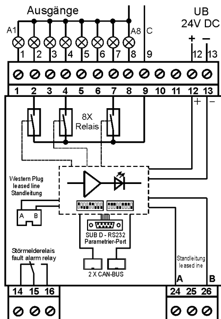
Grundmodul mit Standleitungs-Modem und 8 Ausgangsrelais
